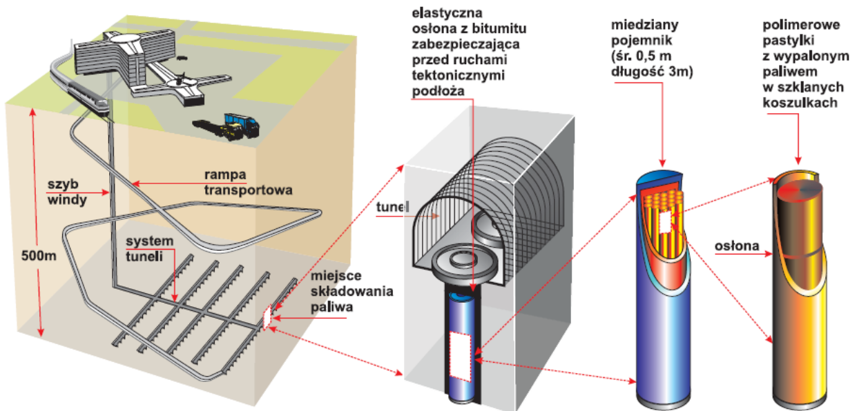
Rys. 2 System barier przy przechowywaniu wypalonego paliwa w Szwecji
